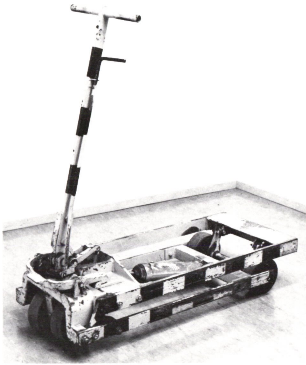
Lågflyt från 1920-talet, använd till lastpallar i trä av den typ som användes före andra världskriget. Efter andra världskriget när ny palltyp infördes användes lågflyften till speciella tryckeripallar i metall. Lågflyften användes vid Postens Centralförråd på 1950-talet. Gåva från Postens Inköpscentral.
